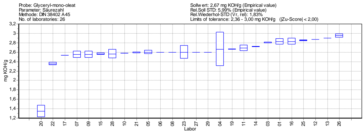
Bild 17. Säurezahl, Graphische Darstellung der Messwerte
